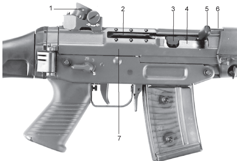
Figure 3 Boîte de culasse
