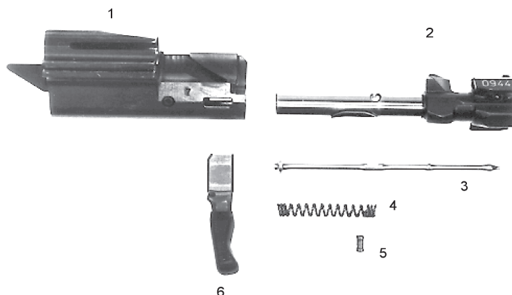
Figure 4: Culasse démontée
