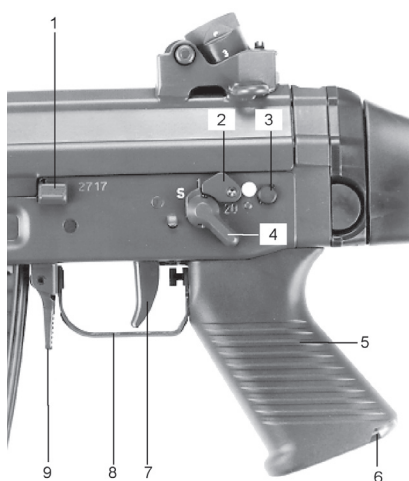
Figure 6: Dispositif de détente
