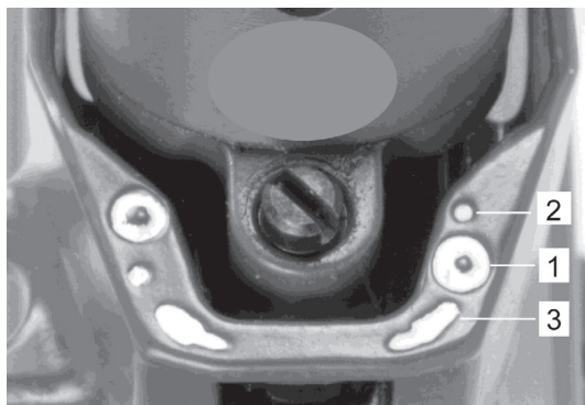
Figure 28: Vis de réglage en élévation
